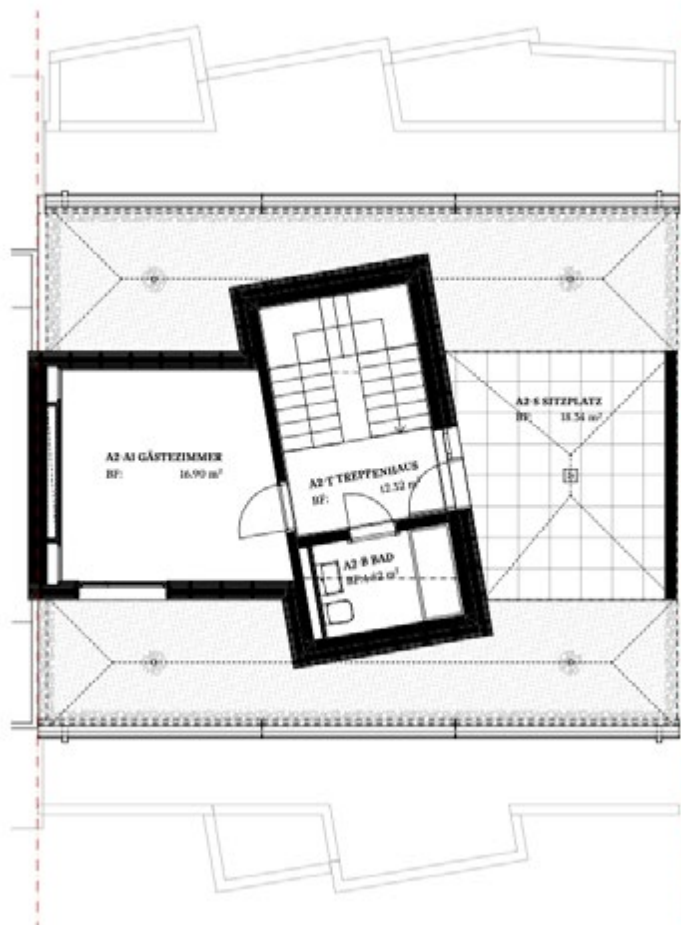
Attikageschoss 2, Dachterrasse mit Gästezimmer und Badezimmer mit Badewanne
