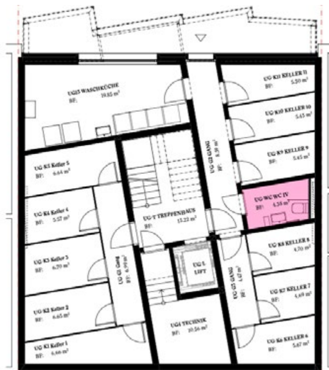
Kellergeschoss (gartenseitig ebenerdig) mit Waschküche und Kellerabteilen
