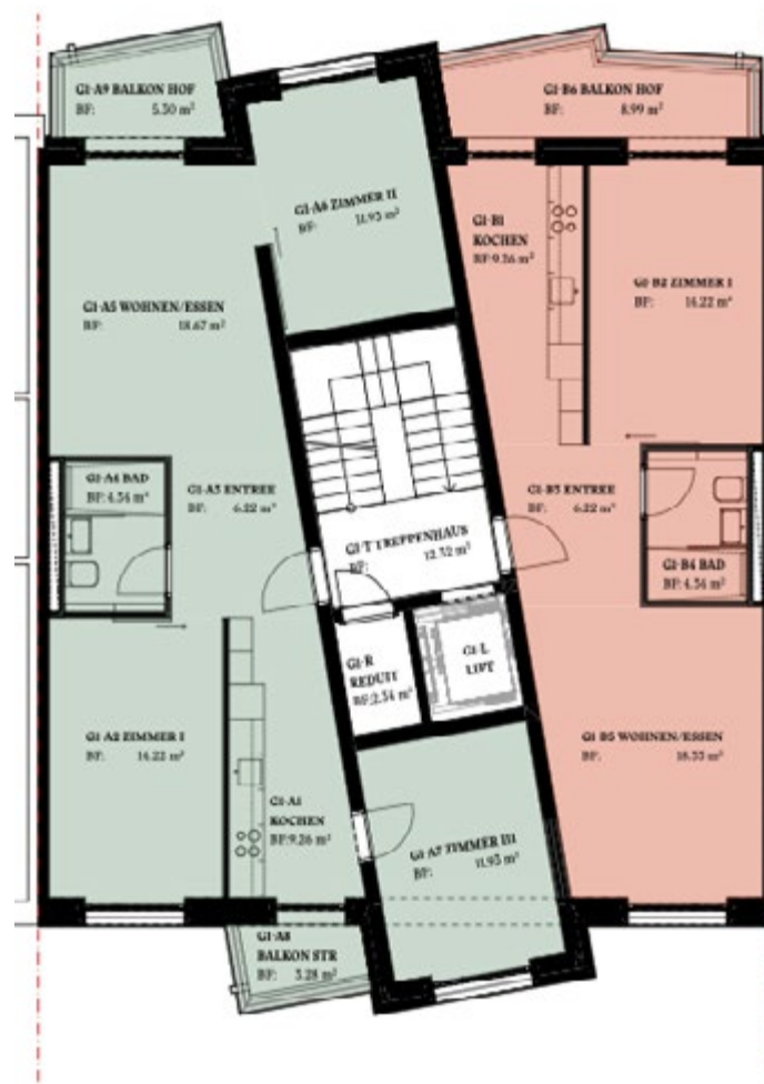
Regelgeschoss, grün eingefärbt eine 4.5 Zimmer-Wohnung, rot eingefärbt eine 2.5 Zimmer-Wohnung
